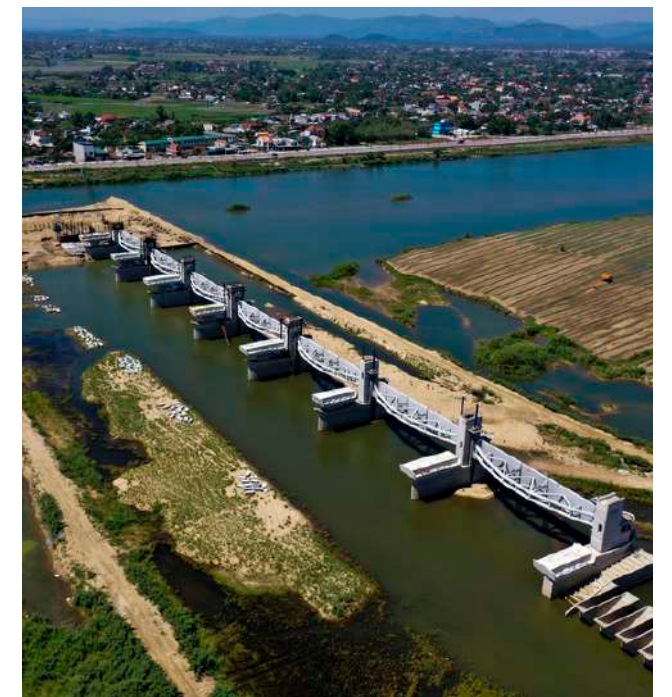
ĐẬP DÂNG HẠ LƯU SÔNG TRÀ KHÚC DAM DOWNSTREAM OF TRA KHUC RIVER
